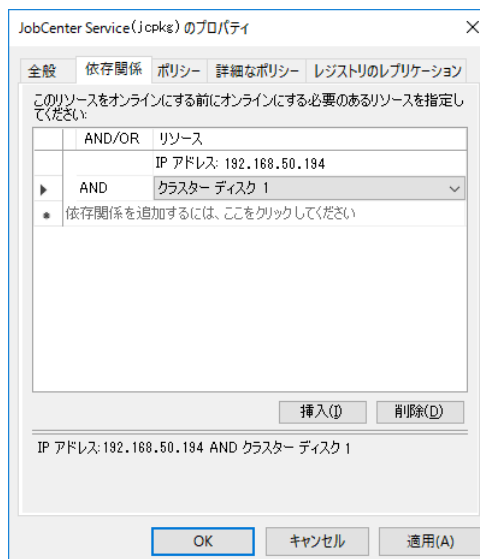
図4.7 依存関係設定画面例
