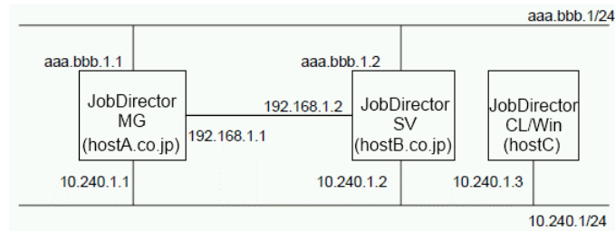
図2.2 IPアドレスの指定例
